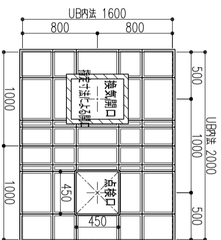
天井パネル外観伏せ図 (S=1/40)
