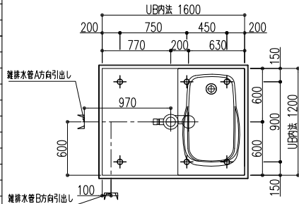
床支持位置:雑排水トラップ芯位置 (S=1/60)
