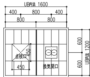
天井パネル外観伏せ図 (S=1/60)
