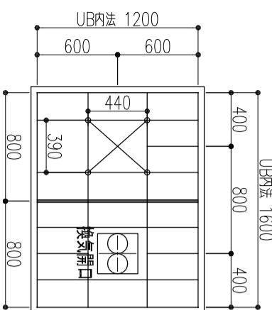
天井パネル外觀伏図
